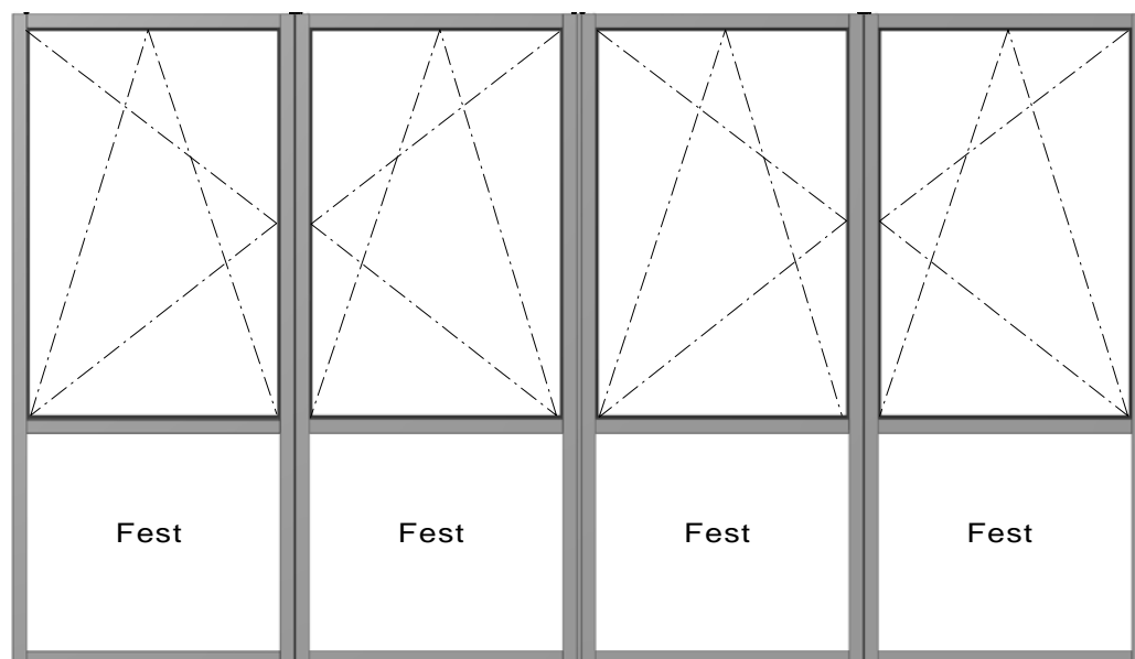
Unterbaulement aus WF-VARIO LUX Integral Glasfläche 11,04 m 2
